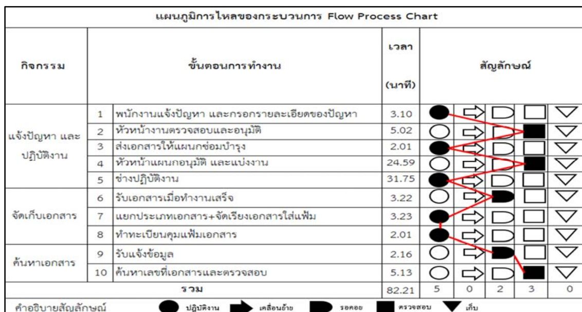
ตารางที่ 5 แผนภูมิกระบวนการไหล ของกิจกรรมการจัดการเอกสาร (หลังปรับปรุง)
