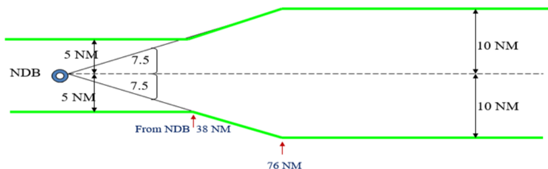
ภาพที่ 2 ขนาดความกว้างของเส้นทางบินซึ่งใช้เครื่องช่วยเดินอากาศแบบ NDB
