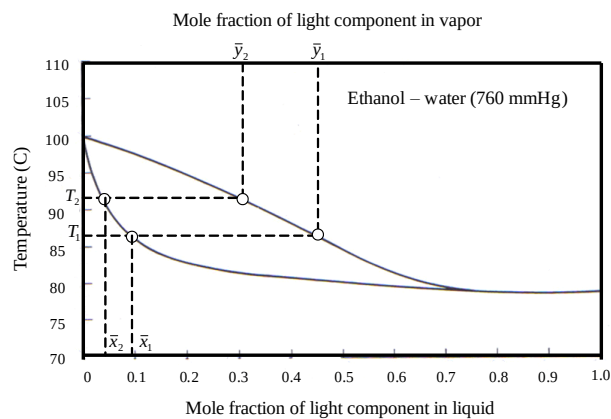
ภาพที่ 1 แผนภาพสมดุลของของผสมไอน้ำ - ของเหลวที่มี 2 องค์ประกอบภายใต้สภาวะความดันคงที่
