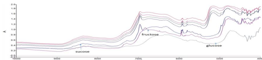
ภาพที่ 4 สเปกตรัมการดูดกลืนแสงของ FT-NIR ที่ช่วงคลื่น 10000 - 4000 \text{cm}^{-1} ของน้ำตาลมะพร้าวแท้ จังหวัดสมุทรสงครามเทียบกับน้ำตาลซูโครส น้ำตาลกลูโคส และน้ำตาลฟรักโตส
