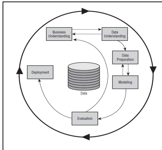
ภาพที่ 1 กระบวนการ CRISP-DM (Jyoti, Nidhi and Sanjeev, 2013)
