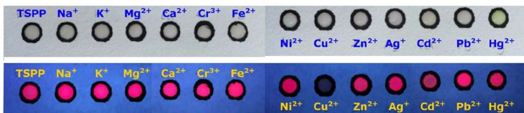
ภาพที่ 6 การทดสอบการเปลี่ยนแปลงทางสีที่สังเกตด้วยตาเปล่าและทางฟลูออเรสเซนซ์แบบกระดาษอย่างง่าย (Prabpal et al., 2017)
