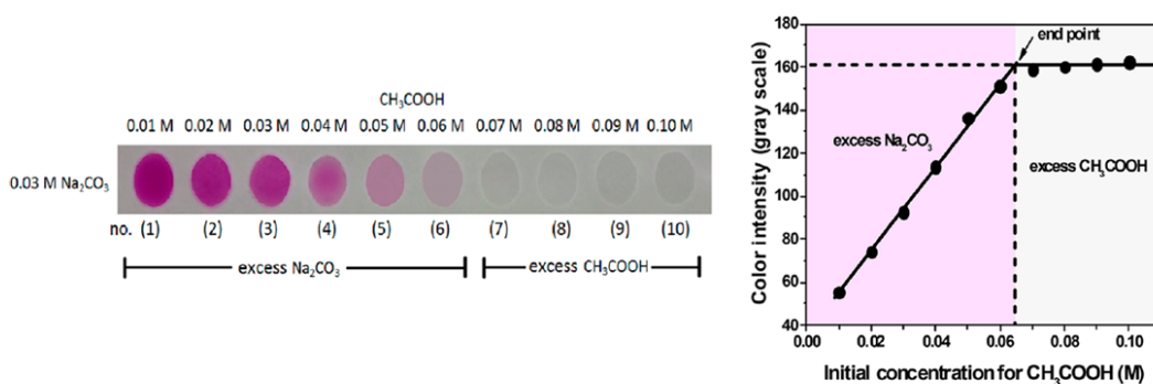
ภาพที่ 8 (ซ้าย) อุปกรณ์แบบกระดาดเพื่อศึกษาสารกำหนดปริมาณจากปฏิกิริยาระหว่าง \text{Na}_2\text{CO}_3 กับ \text{CH}_3\text{COOH} ; (ขวา) การวิเคราะห์เชิงปริมาณโดยการวิเคราะห์ความเข้มของสี (สีเทา) ด้วยโปรแกรม ImageJ (Namwong et al., 2018)
