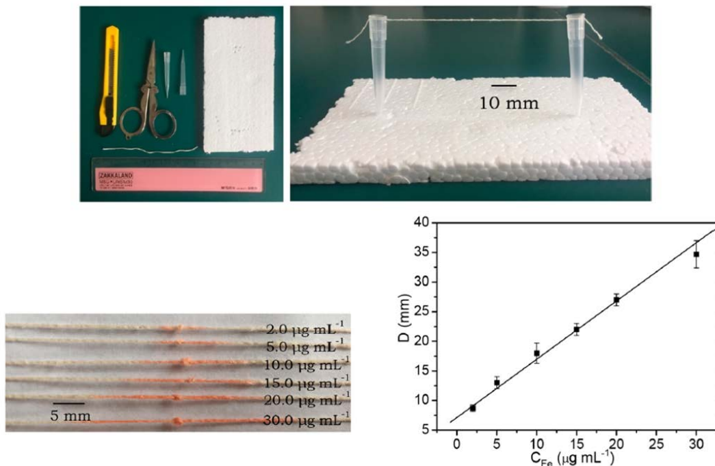
ภาพที่ 12 (บน) วัสดุที่จำเป็นสำหรับการสร้างอุปกรณ์ตรวจวิเคราะห์ไมโครฟลูอิดิกส์เส้นด้ายด้วยการวัดระยะทาง และตัวอย่างการติดตั้งอุปกรณ์สาธิตการทดลอง; (ล่าง) แถบสีบนเส้นด้ายและกราฟมาตรฐานที่พล็อตระหว่างความเข้มข้นของ \text{Fe}^{2+} กับระยะที่วัดได้ (Cai et al., 2019)
