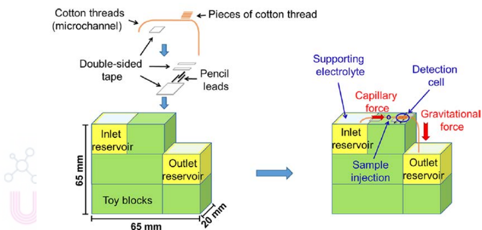
ภาพที่ 11 (ซ้าย) วัสดุที่นำมาสร้างอุปกรณ์วิเคราะห์ทางเคมีไฟฟ้าไมโครฟลูอิดิกส์ และ (ขวา) หลักการทำงานอาศัยอาศัยแรงแคปิลลารีควบคู่กับแรงโน้มถ่วงของโลก (Xu et al., 2018)
