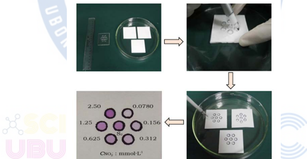
ภาพที่ 3 สร้างชุดการทดลองไมโครฟลูอิดิกส์แบบกระดาษด้วยปากกามาร์คเกอร์เคมีชนิดถาวรเพื่อใช้หาปริมาณไนเตรตไอออน ( \text{NO}_2^- ) (Wang et al., 2015)
