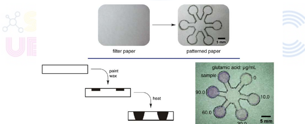
ภาพที่ 1 (บน) โชนวงกลมออกเป็น 6 แฉกบนกระดาษกรอง; (ล่าง) ขี้ผึ้งละลายและซึมเข้าสู่กระดาษเพื่อตรวจหาปริมาณกรดอะมิโนในสารสกัดจากชาด้วยสารละลายนินไฮดริน (Cai et al., 2012)
