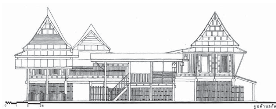
รูป 5 เปรียบเทียบรูปด้านหน้า บน: เรือนของคนไทยพื้นถิ่น กลาง: เรือนของคนกลุ่มชาติพันธุ์จีน ล่าง: เรือนของคนกลุ่มชาติพันธุ์มุสลิม
