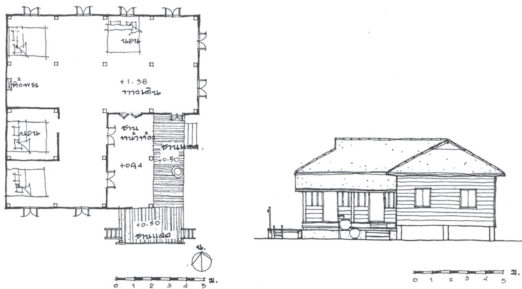
ภาพที่ 14: แผนผังและรูปด้านเรือนมุข บ้านกลาง อำเภอยางชุมน้อย จังหวัดเลย ที่มา: ทรงยศและคณะ, 2548
