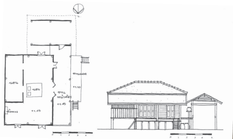
ภาพที่ 12: แผนผังและรูปด้าน เรือนหลังคาบ้านหยาบกระเบื้องซีเมนต์ บ้านกลาง อำเภอยางชุมน้อย จังหวัดเลย ที่มา: ทรงยศและคณะ, 2548
