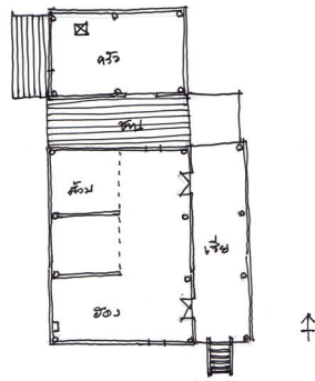
ภาพที่ 5: แผนผังเรือนเกาะเดี่ยวตามคำบอกเล่าของชาวบ้านกลาง
