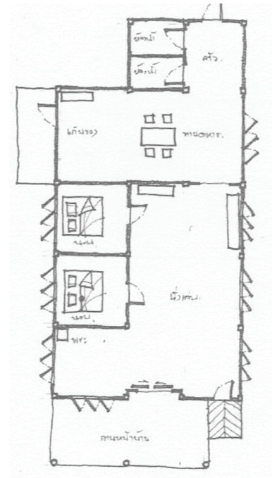
ภาพที่ 22: แผนผัง เรือนบ้านชั้นเดียว บ้านกลาง ที่มา: นพดล ตั้งสกุล และคณะ, 2553
