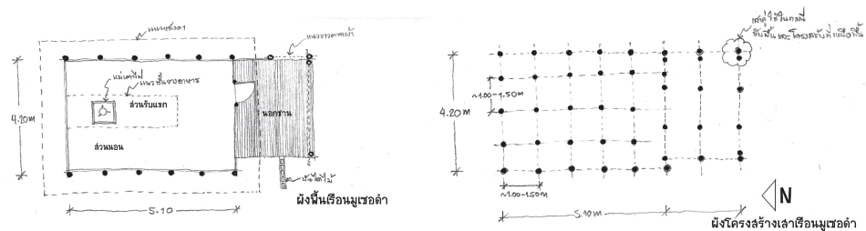
ภาพที่ 6: ผังเรือนและโครงสร้างเสาเรือนลาหู่ จังหวัดตาก (หน่วยเป็นเมตร)
