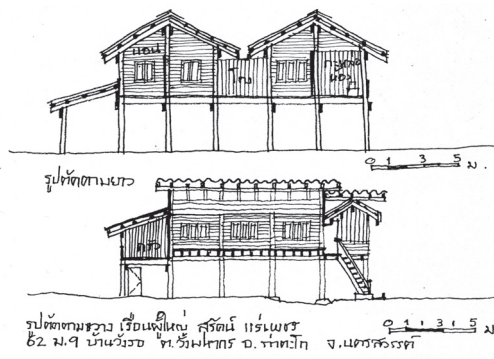
ภาพที่ 3: ผังพื้นชั้นบน รูปตัดตามยาว และรูปตัดตามขวาง เรือนผู้ใหญ่สุรัตน์ แร่เพชร 62 หมู่ 9 บ้าน วังรอง ตำบลวังมหาร อำเภท่าตะโก จังหวัดนครสวรรค์
