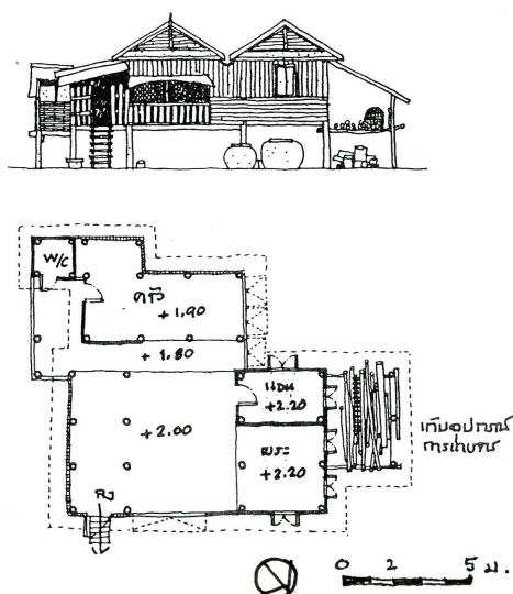
ภาพที่ 14: รูปด้าน และ ผังพื้นชั้นบน ของเรือนที่สำรวจ เมื่อเดือน มีนาคม 2544 เรือน นางบุญเสริม กุณาหน ที่ผังพื้นเรือนยังเหมือนเดิมทุกประการ
