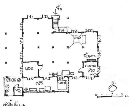
ภาพที่ 3: ผังพื้นชั้นบน รูปตัดตามยาว และรูปตัดตามขวาง เรือนผู้ใหญ่สุรัตน์ แร่เพชร 62 หมู่ 9 บ้าน วังรอง ตำบลวังมหาร อำเภท่าตะโก จังหวัดนครสวรรค์
