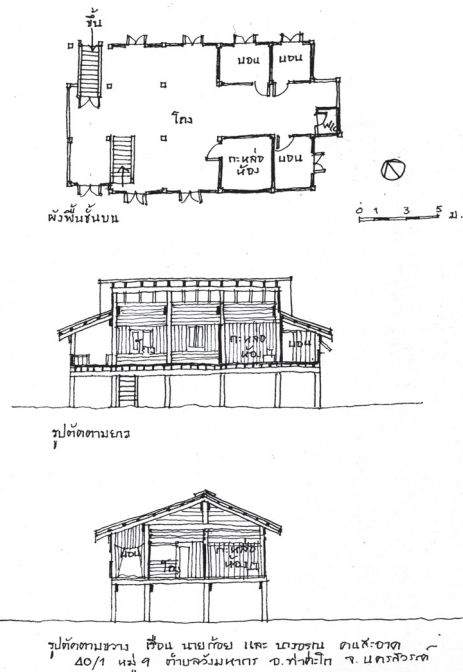
ภาพที่ 8: ผังพื้น รูปตัดตามยาว และรูปตัดตามขวาง เรือนนายก่อย และนางอรุณ คนสะอาด 40/1 หมู่ 9 บ้านวังร่อ ตำบลวังมหากกร อำเภอทาดะโก จังหวัดนครสวรรค์
