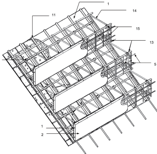
ภาพที่ 11: แสดงวิธีติดตั้งแผ่น “คอนกรีตเสริมเหล็กพร้อมเหล็กเสริม” ที่ใช้เป็นบันไดด้วยรูปตัดทัศนียภาพ
