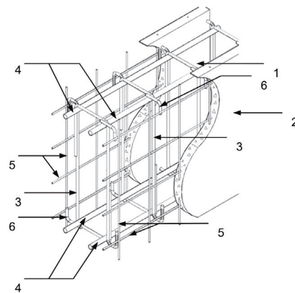
ภาพที่ 2: แสดงวิธีการติดตั้งแผ่น “คอนกรีตเสริมเหล็กพร้อมเหล็กเสริม” ในการใช้เป็นคานด้วยรูปตัดทัศนียภาพ
