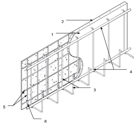
ภาพที่ 1: แสดงรูปตัดทัศนียภาพของแผ่น “คอนกรีตเสริมเหล็กพร้อมเหล็กเสริม” ที่ใช้เป็นคาน
