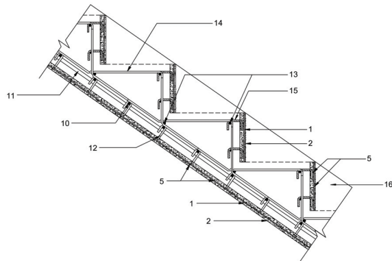
ภาพที่ 8: แสดงวิธีติดตั้งแผ่น “คอนกรีตเสริมเหล็กพร้อมเหล็กเสริม” ที่ใช้เป็นบันไดด้วยรูปตัดตามขวาง
