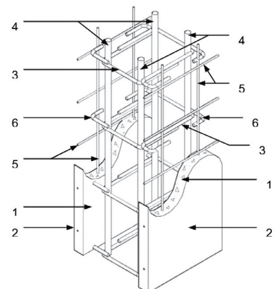
ภาพที่ 4: แสดงวิธีการติดตั้งแผ่น “คอนกรีตเสริมเหล็กพร้อมเหล็กเสริม” ในการใช้เป็นเสาด้วยรูปตัดทัศนียภาพ
