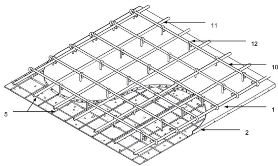
ภาพที่ 9: แสดงรูปทัศนียภาพของแผ่น “คอนกรีตเสริมเหล็กพร้อมเหล็กเสริม” ที่ใช้เป็นท้องพื้นบันได
