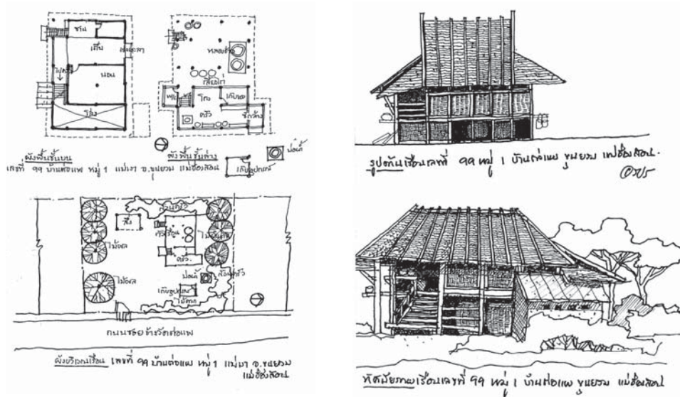
ภาพที่ 7: ผังบริเวณ ผังพื้น และรูปลักษณะของเรือนไทใหญ่ บ้านต่อแพ อำเภอขุนยวม จังหวัดแม่ฮ่องสอน
