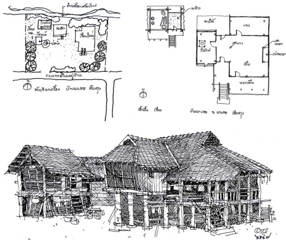
ภาพที่ 9: ผังบริเวณ ผังพื้น และรูปลักษณะของเรือนไทใหญ่ที่บ้านยางลอ เชียงตุง เมียนมาร์
