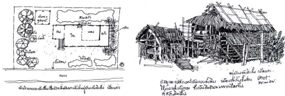
ภาพที่ 12: ผังบริเวณ ผังพื้นและรูปลักษณะของเรือนไทใหญ่แบบดั้งเดิม หมู่บ้านต้าเต็งฮั่น เมืองมว แคว้นไตคอง สาธารณรัฐประชาชนจีน
