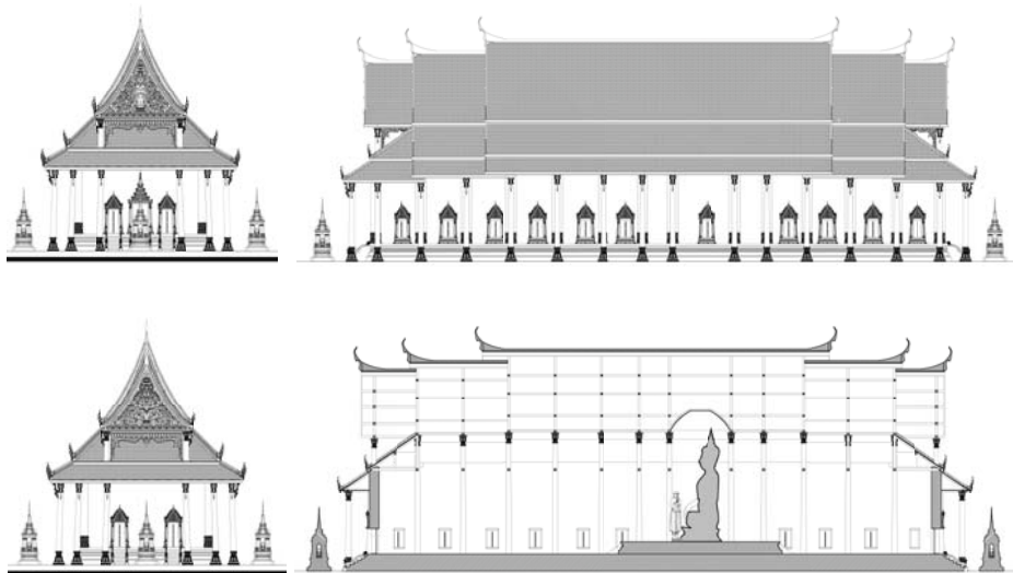
ภาพที่ 23: แบบสถาปัตยกรรมพระวิหารหลวงวัดพระบรมธาตุนครธรรมราชซึ่งออกแบบเป็นอาคาร ขนาดใหญ่ และมีหลังคามุขประเจิดที่มีความงดงามอย่างยิ่ง (บนซ้าย) รูปด้านหน้า (บนขวา) รูปด้านข้าง แลเห็นส่วนที่เป็นมุขประเจิด (ล่างซ้าย) รูปตัดขวาง (ล่างขวา) รูปตัดตามยาว
