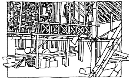
พื้นที่ครัว เตา: ผนังจาก ดินเหนียว เหนียวเพื่อ เก็บไฟไม่ให้ ลุกลาม
