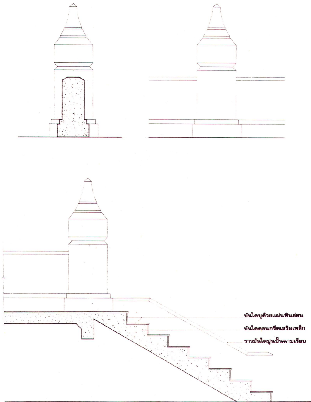
แบบขยาย (รูปตัดบันได ราวระเบียง)
