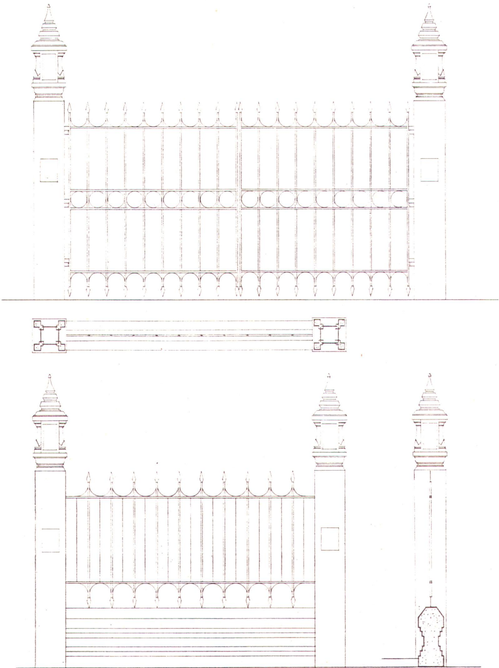
แบบขยายรั้ว
