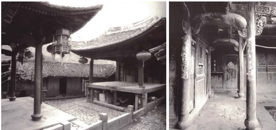
ภาพที่ 1: แสดงการตั้งเสาไม้บนก้อนหินของสถาปัตยกรรมพื้นถิ่นจีน
