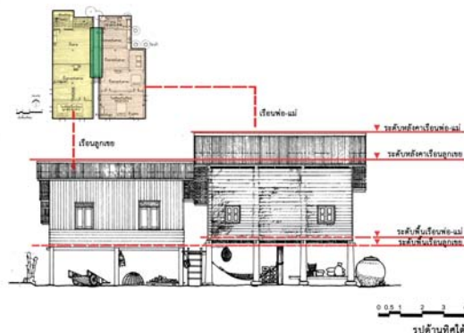
ภาพที่ 13: เรือนกรณีศึกษาที่ 5 แสดงระดับสูง-ต่ำ ของเรือนลูกเขยกับเรือนพ่อแม่ จะเห็นว่าเรือนที่ปลูกสร้างใหม่จะลดระดับของพื้นและหลังคาให้ต่ำกว่าเรือนเดิมของพ่อแม่
