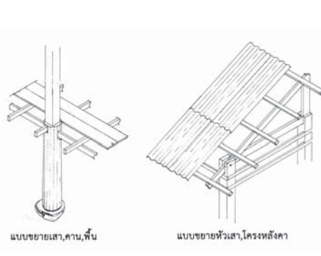
ภาพที่ 11: แสดงแบบขยายเสาและโครงหลังคาเรือนเสาที่วางตั้งบนก้อนหิน
