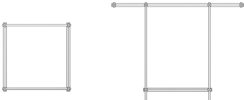
ภาพที่ 10: ผังพื้น (ซ้าย) และรูปด้าน (ขวา) ของศาลาต้นแบบ
