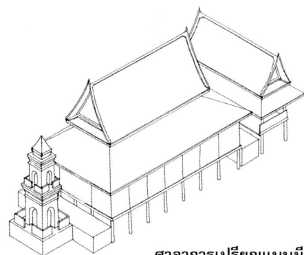
ศาลาการเปรียญแบบมีหอรอง ด้านหน้า ศาลาขวางด้านหลัง
