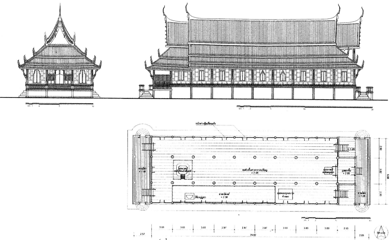
ผังพื้น รูปตั้งด้านหน้าและด้านข้าง ศาลาการเปรียญวัดใหญ่สุวรรณาราม
