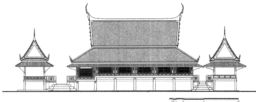
ผังพื้น รูปตั้งด้านหน้าและด้านข้าง ศาลาการเปรียญวัดเกาะแก้วสุทธาราม
