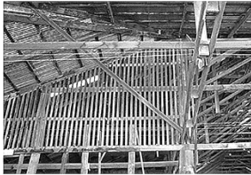
บริเวณแผงข้างใน
