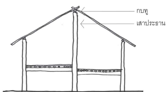
รูปที่ 6 จั่วเรือนที่กบทุวางบนเสาดั้ง (ซ้าย) และจั่วเรือนที่กบทุวางบนเสาประธาน (ขวา) ที่มา: รวบรวมข้อมูลโดยผู้วิจัย
