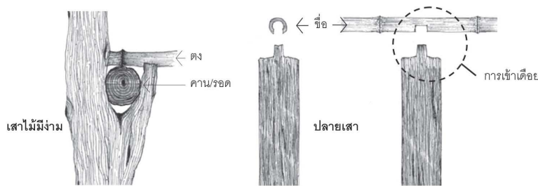
รูปที่ 13 แสดงการใช้เสามาที่มีง่ามเพื่อรองรับคานหรือรอด (ซ้าย) การเข้าไม้ด้วยการเหลาเป็นเดือยและเสียบ (ขวา)
