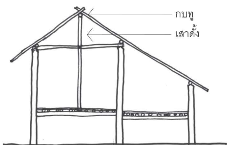
รูปที่ 6 จั่วเรือนที่กบทุวางบนเสาดั้ง (ซ้าย) และจั่วเรือนที่กบทุวางบนเสาประธาน (ขวา) ที่มา: รวบรวมข้อมูลโดยผู้วิจัย
