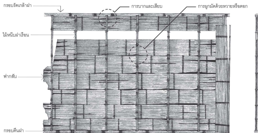
รูปที่ 15 แสดงการเข้าไม้ส่วนฝาเรือนด้วยการใช้โครงไม้ไผ่หนีบฟากสับยึดด้วยการบากและเสียบ ร่วมกับการผูกมัดด้วยหวาย/ตอก
