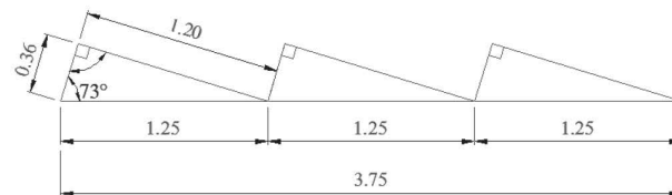
รูปที่ 9 แสดงรายละเอียดระยะของ crib สะท้อนเสียงทางด้านข้างของห้องบรรยาย
