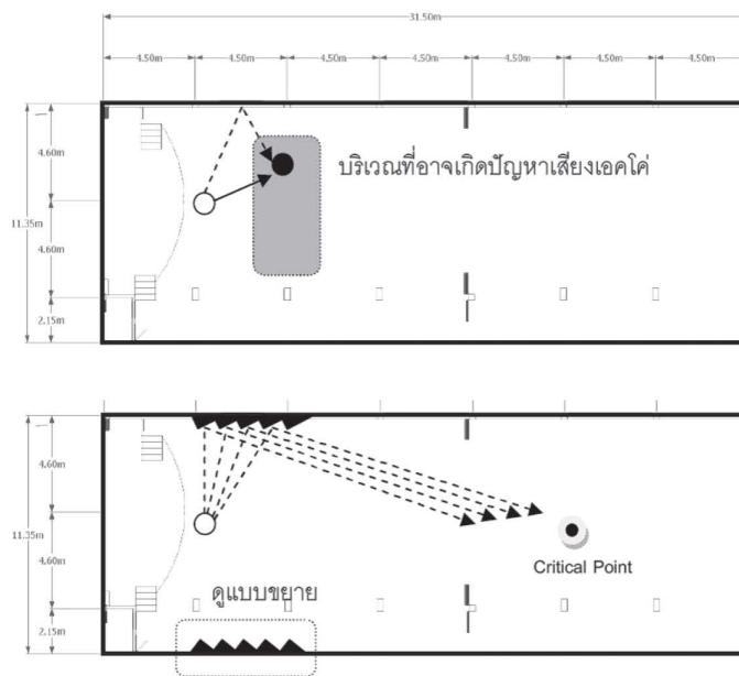
รูปที่ 8 แสดงการแก้ปัญหาเสียงสะท้อนหรือเสียงเอคโคโดยใช้ crib สะท้อนเสียงด้านข้างเพื่อกระจายเสียงไปยังจุดที่มักจะไม่ได้ยินเสียงบรรยายคือจุดกึ่งกลางห้องจากด้านหลังระยะ 1 ใน 3 ของห้อง (Critical Point) (สุนทร บุญญาธิการ, 2545) และเพื่อแก้ปัญหาเสียงเอคโคบริเวณแถวหน้า
