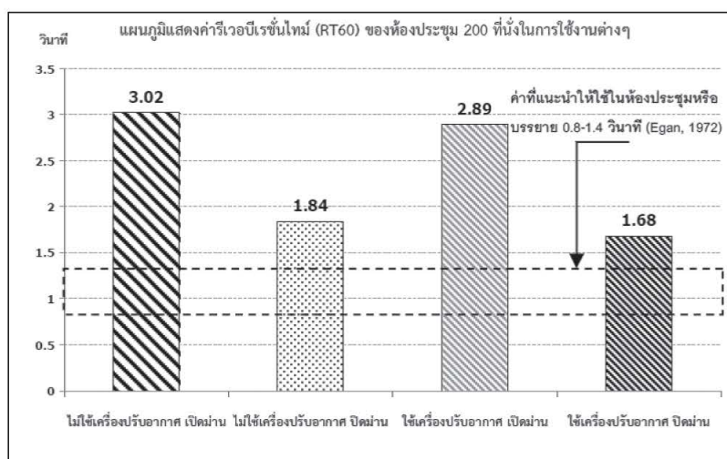
แผนภูมิที่ 2 แสดงค่าเฉลี่ยของรีเวอร์เบชันไทม์ (RT60) หน่วยเป็นวินาที ของห้องบรรยายขนาด 200 ที่นั่ง
