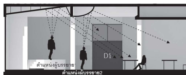
รูปที่ 10 แสดงรายละเอียดของฝ้าเพดานสะท้อนเสียงทางด้านบนเพดานของห้องบรรยาย
