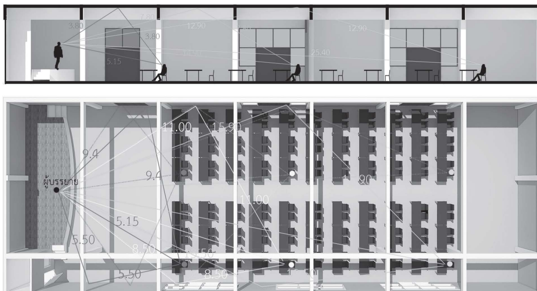
รูปที่ 4 แสดงการวิเคราะห์การเกิดเอคโคของเสียงโดยวิธี Ray Analysis ของห้องบรรยายและประชุมขนาด 200 ที่นั่ง โดยการพิจารณาตำแหน่งของผู้ฟัง 6 จุด ได้แก่ หน้าห้องกลางแถว หน้าห้องริมแถว กลางห้องกลางแถว กลางห้องริมแถว หลังห้องกลางแถว และกลางห้องริมแถว โดยการสะท้อนจากผนังและฝ้าเพดาน
