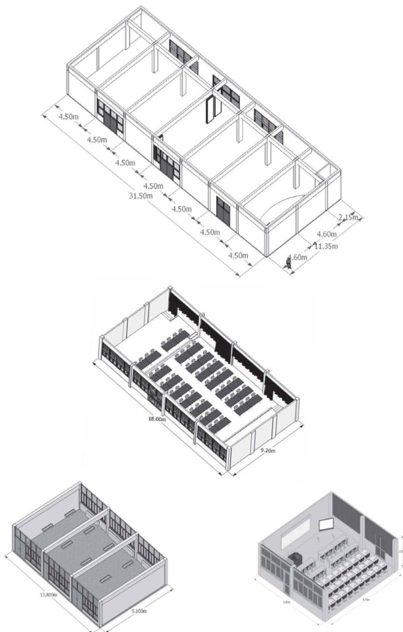
รูปที่ 3 แสดงลักษณะทางกายภาพของห้องบรรยายขนาดต่างๆ ได้แก่ห้องบรรยายขนาด 200 ที่นั่ง (บน) 100 ที่นั่ง (กลาง) 50 ที่นั่ง (ล่างซ้าย) และ 30 ที่นั่ง (ล่างขวา)
