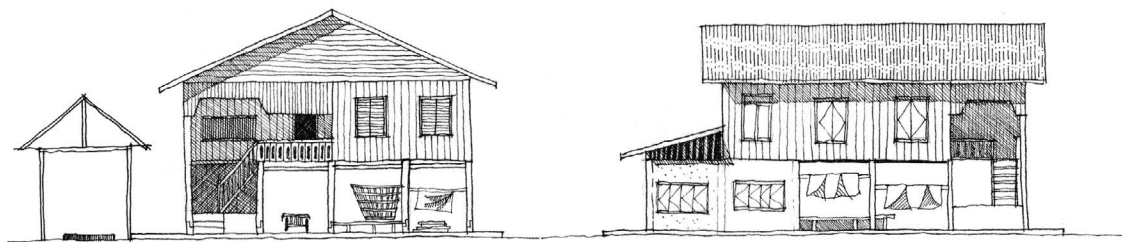
รูปที่ 4 แบบเรือนไทใหญ่แบบประยุกต์ บ้านต่อแพ อำเภอขุนยวม จังหวัดแม่ฮ่องสอน ที่มา: จากการเก็บข้อมูลภาคสนาม
