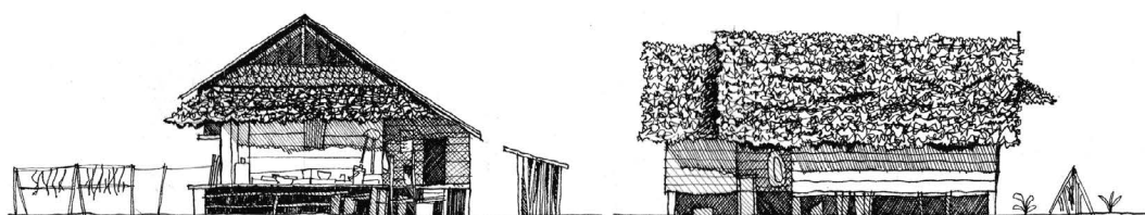
รูปที่ 2 แบบเรือนไทใหญ่แบบจั่วเดี่ยว บ้านต่อแพ อำเภอขุนยวม จังหวัดแม่ฮ่องสอน ที่มา: จากการเก็บข้อมูลภาคสนาม
