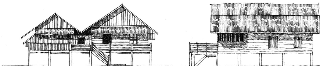
รูปที่ 3 แบบเรือนไทใหญ่แบบสองจั่ว บ้านต่อแพ อำเภอขุนยวม จังหวัดแม่ฮ่องสอน ที่มา: จากการเก็บข้อมูลภาคสนาม
