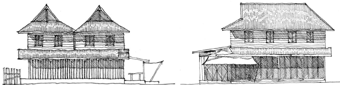
รูปที่ 5 แบบเรือนไทใหญ่แบบเรือนร้านค้า พื้นที่ชุมชนขุนยวม อำเภอขุนยวม จังหวัดแม่ฮ่องสอน ที่มา: จากการเก็บข้อมูลภาคสนาม
