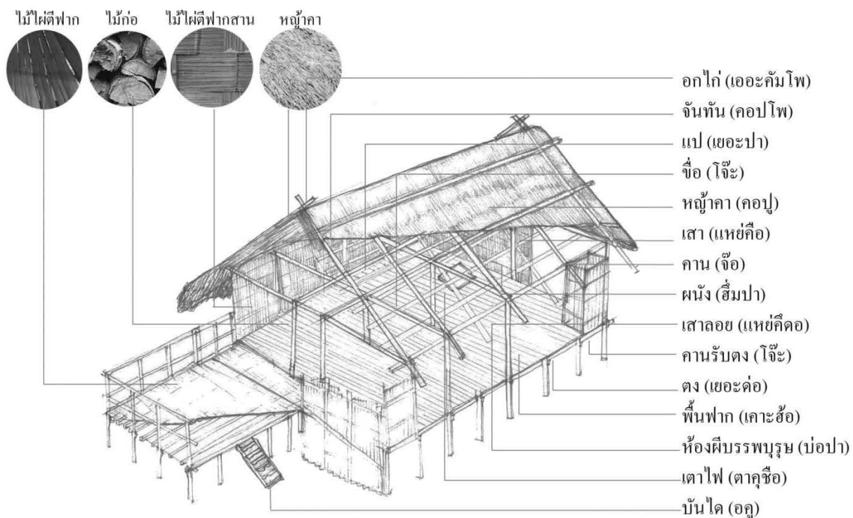
รูปที่ 5 ส่วนประกอบและโครงสร้างเรือนดั้งเดิม (สำรวจเมื่อปี พ.ศ. 2556-2557) ที่มา: รวบรวมข้อมูลโดยผู้วิจัย
