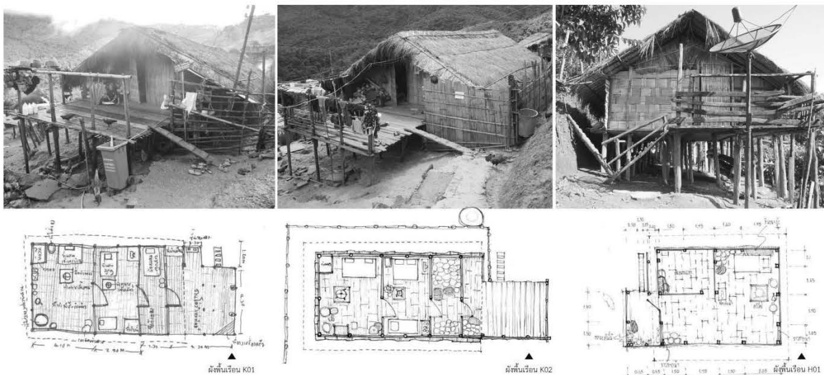
รูปที่ 6 รูปแบบและผังพื้นเรือนดั้งเดิม (สำรวจเมื่อปี พ.ศ. 2556-2557) ที่มา: รวบรวมข้อมูลโดยผู้วิจัย
