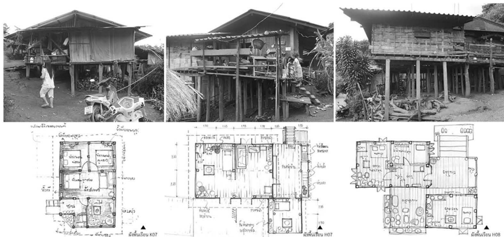
รูปที่ 8 รูปแบบและผังพื้นเรือนต่อเติม (สำรวจเมื่อปี พ.ศ. 2556-2557)
