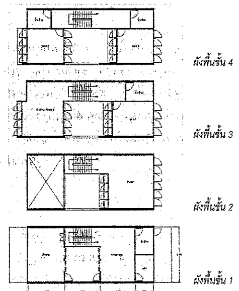
รูปที่ 12 ผังพื้นอาคารตีกรวแบบทงเลือกที่ 3
