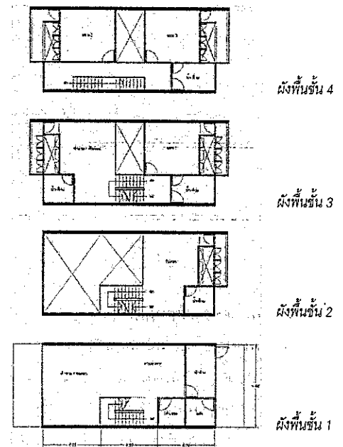
รูปที่ 8 ผังพื้นอาคารตีกรวแบบทงเลือกที่ 2
