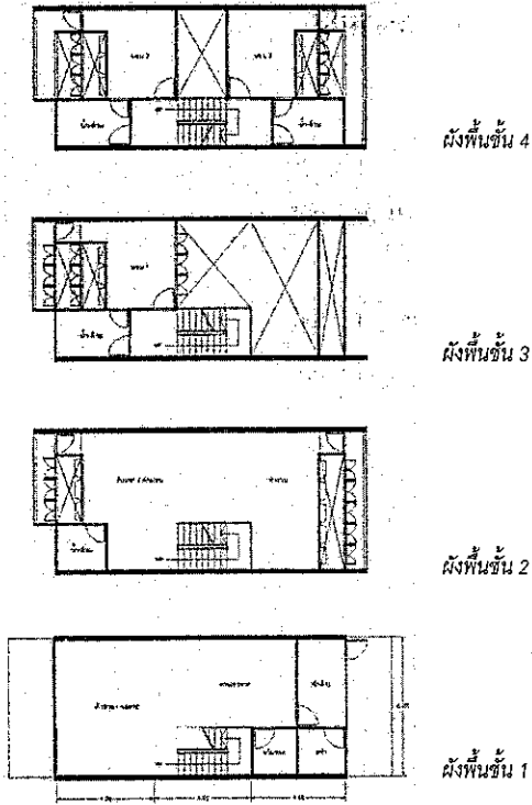
รูปที่ 4 ผังพื้นอาคารติดแนวแบบทางเลือกที่ 1
