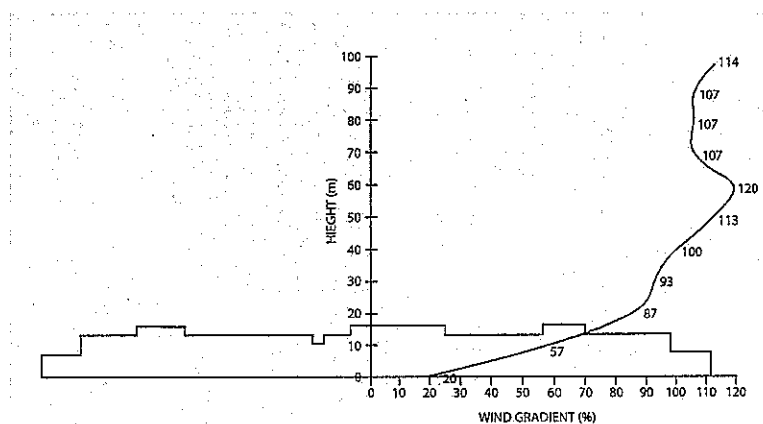
รูปที่ 3 แผนภาพแสดงความเร็วลมที่วัดได้ (%) ณ ระดับความสูงทุก 10 เมตร จากหุ่นจำลองบริเวณเขตหน่วยขวาง
