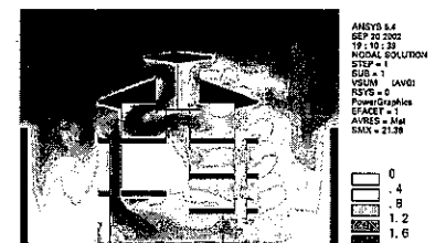
รูปที่ 11 ผลการทดลองด้วยคอมพิวเตอร์ แสดงความเร็วลมภายในอาคาร ตีกรวแบบทงเลือกที่ 2 กรณีกที่ 3
