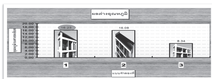
รูปที่ 7 แสดงแผนภูมิสรุปผลค่าความแตกต่างของอุณหภูมิกายนอกกับภายในของแบบจำลองทั้งสาม ที่มา: (แผนภูมิภาพนี้ผู้วิจัยได้จัดทำขึ้นเพื่อสรุปผลค่าความแตกต่างของอุณหภูมิกายนอกกับภายในของแบบจำลองสำหรับงานวิจัยนี้)
