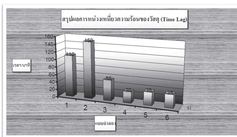
รูปที่ 8 แสดงแผนภูมิสรุปผลค่าการหน่วงเหนี่ยวความร้อนของวัตถุ (Time Lag) ในของแต่ละแบบจำลองทั้งสาม ที่มา: (แผนภูมิภาพนี้ผู้วิจัยได้จัดทำขึ้นเพื่อสรุปผลค่าการหน่วงเหนี่ยวความร้อนของวัตถุ (T ในของแต่ละแบบจำลองสำหรับงานวิจัยนี้)
