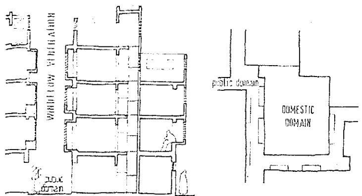
รูปที่ 9 แสดงภาพตัดขวางบ้านแบบ High-rise street frontage housing [ที่มา (2) หน้า 371]
