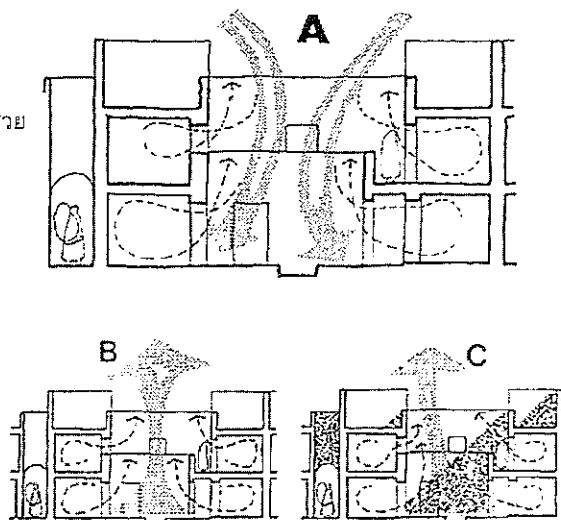
รูปที่ 2 แสดงภาพตัดขวางบ้านแบบ Courtyard housing มักก่อสร้างด้วยกำแพงทึบตัน มีช่องเปิดน้อย หลังคาหนา เพื่อลดความร้อนภายในอาคาร [ที่มา (2) หน้า 370]
