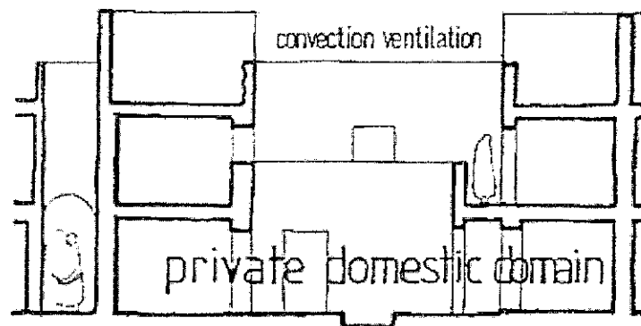
รูปที่ 2 แสดงภาพตัดขวางบ้านแบบ Courtyard housing มักก่อสร้างด้วยกำแพงทึบตัน มีช่องเปิดน้อย หลังคาหนา เพื่อลดความร้อนภายในอาคาร [ที่มา (2) หน้า 370]
