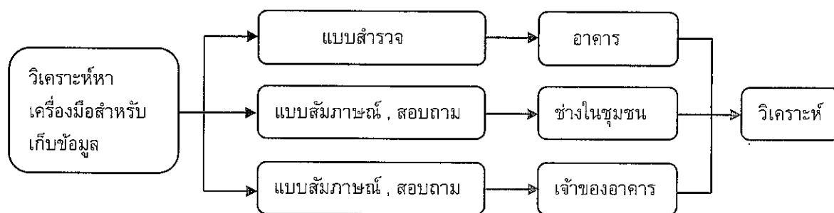
รูปที่ 2 แสดงวิธีการวิเคราะห์หารูปแบบเทคโนโลยีการก่อสร้าง
