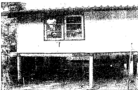
รูปที่ 8 แสดงตอม่อและฐานรากเทคอนกรีตในท่อคอนกรีต
