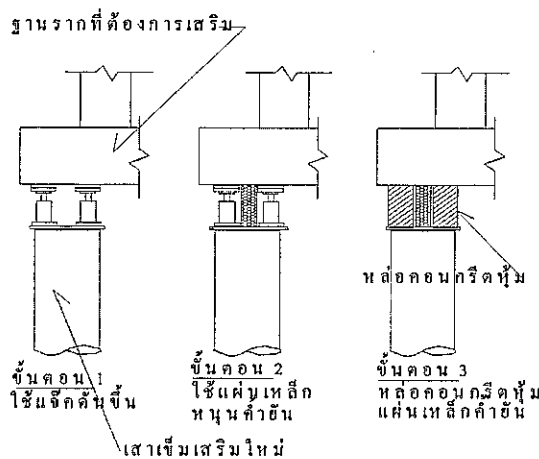
รูปที่ 2 การถ่ายน้ำหนักลงเสาเข็มใหม่
