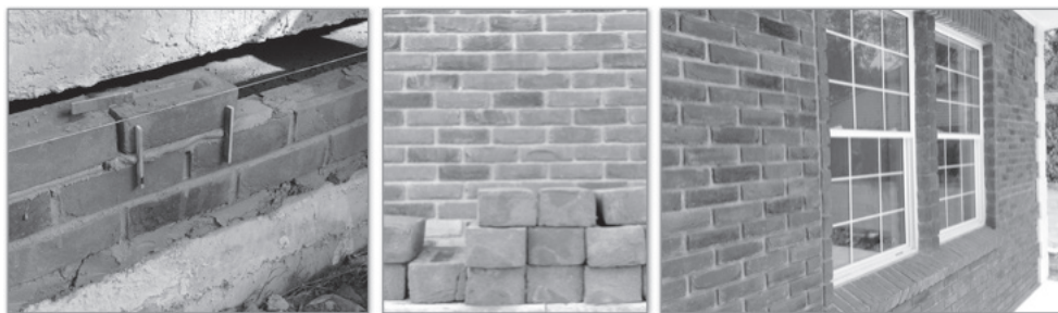
รูปที่ 5 จากซ้าย การเรียงอิฐที่ละก้อนต้องใช้การวัดระดับที่ดี ขนาดของอิฐที่มีความหนา และการใส่รายละเอียดช่องเปิดของหน้าต่าง เช่น วงกบหน้าต่างต้องเอียงก่อนอิฐออกเพื่อการระบายน้ำที่ดี ที่มา: ผู้วิจัย (2558)
