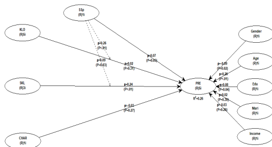
ภาพที่ 3.1: Model 5 Modified Structural Model
