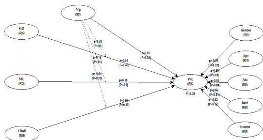
ภาพที่ 3.2 : Model 6 Hypothesized Structural Model for Hypothesis Testing
