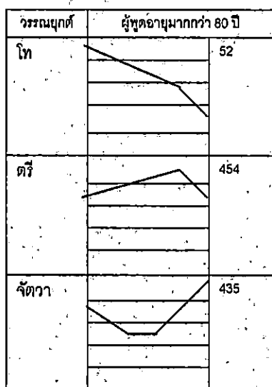
ภาพที่ 10 เปรียบเทียบสัทลักษณะของวรรณยุกต์โท ตรี จัตวา ในผู้พูด 3 กลุ่มอายุ
