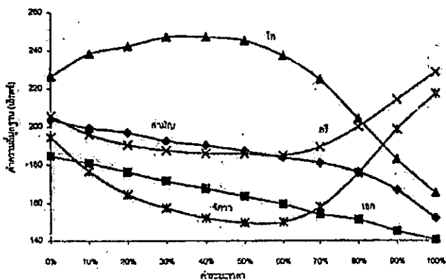
ภาพที่ 5 สัทลักษณะของวรรณยุกต์ภาษาไทยปี ค.ศ. 2000 (จิไลลักษณ์)
