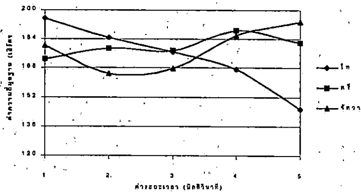
ภาพที่ 6 สัทลักษณะของวรรณยุกต์โท ตรี และจัตวาในผู้พูดอายุมากกว่า 80 ปี
