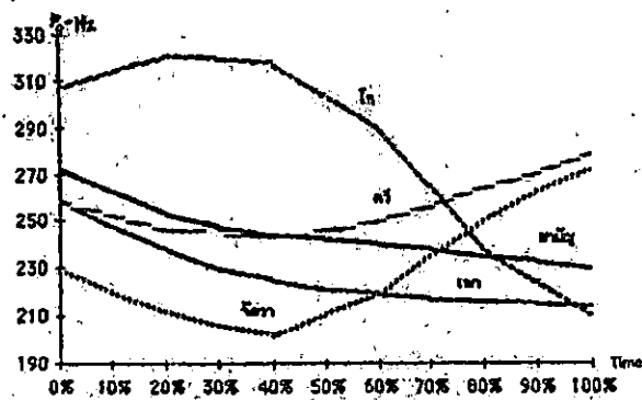
ภาพที่ 2 สัทลักษณะของวรรณยุกต์ภาษาไทยปี ค.ศ. 1991 (ปิยจิตร)
