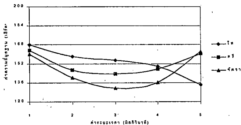
ภาพที่ 8 สัทลักษณะของวรรณยุกต์โท ตี และจิตวาในผู้พูดอายุต่ำกว่า 15 ปี
