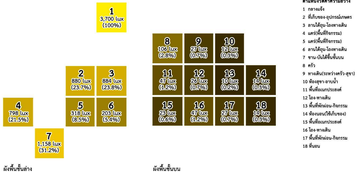
ภาพที่ 6 ค่าความสว่างในตำแหน่งพื้นที่ใช้งานต่าง ๆ และสัดส่วนความสว่างเมื่อเปรียบเทียบกับปริมาณแสงจากภายนอก
