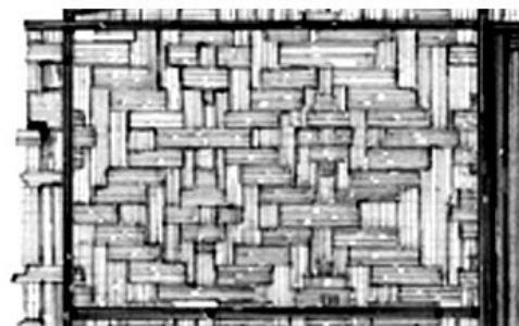
ฝาไม้ไผ่สาน ลมผ่านได้ไม่เกินร้อยละ 2
