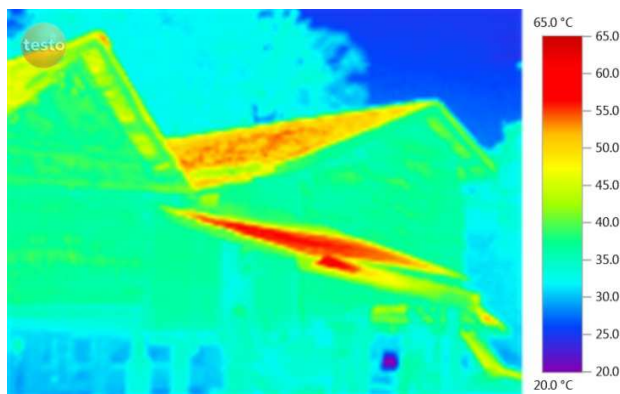
ภาพที่ 2 ภาพเรือนกรณีศึกษา ที่ถ่ายด้วยกล้องถ่ายภาพความร้อนเพื่อเปรียบเทียบอุณหภูมิพื้นผิววัสดุอาคารประเภทต่างๆ
