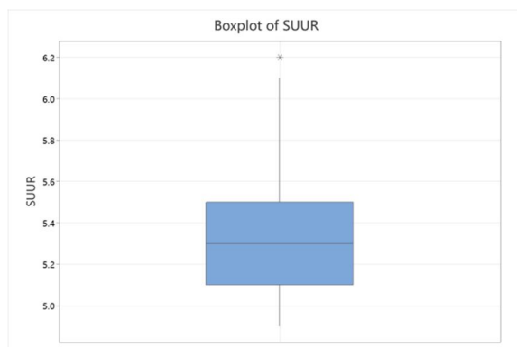
ภาพที่ 2 กราฟบล็อกพล็อต (Box Plot) โปรแกรม Minitab 16
