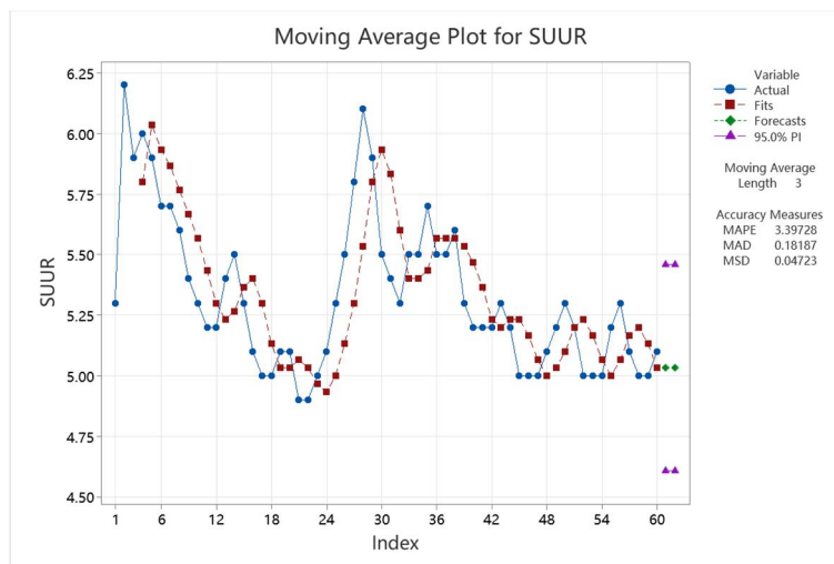
ภาพที่ 7 Moving Average Plot โปรแกรม Minitab 16
