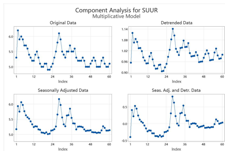
ภาพที่ 5 Component Analysis โปรแกรม Minitab 16
