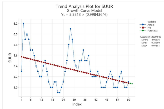
ภาพที่ 3 Trend Analysis Plot โปรแกรม Minitab 16
