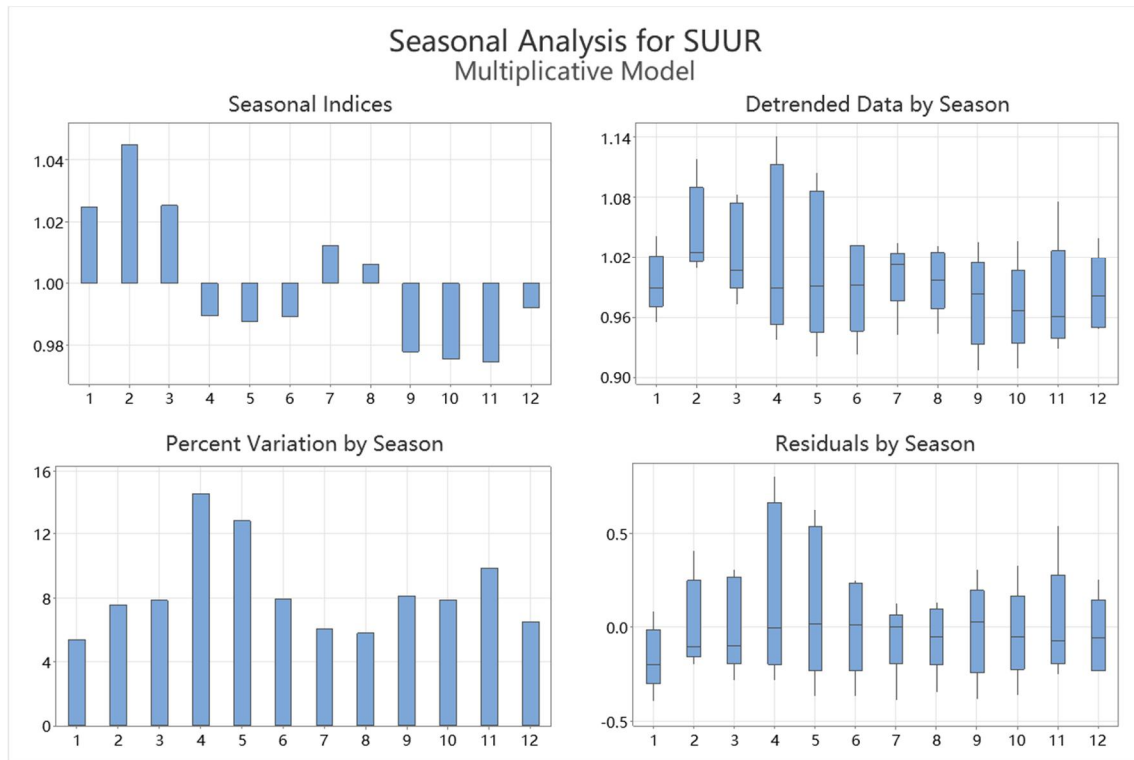
ภาพที่ 6 Seasonal Analysis โปรแกรม Minitab 16
