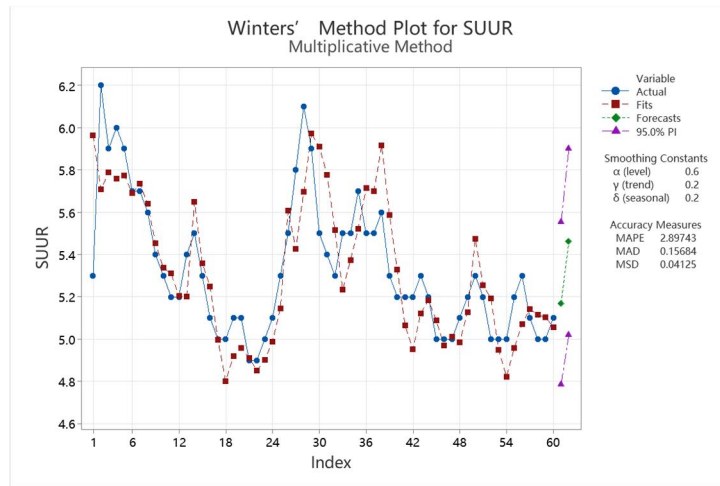
ภาพที่ 10 Winters' Method โปรแกรม Minitab 16
