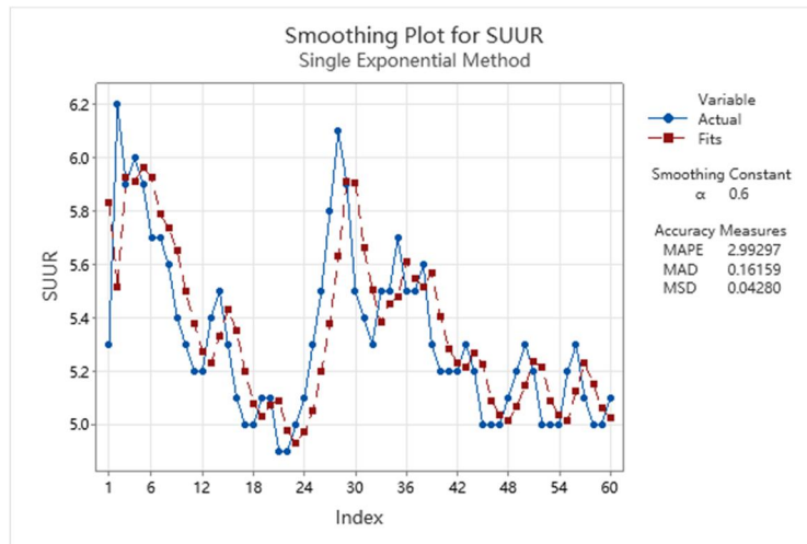
ภาพที่ 8 Single Exponential Method โปรแกรม Minitab 16 ที่มา: Guoxiang (2024)
