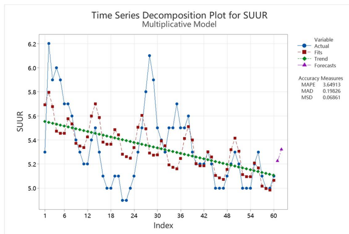
ภาพที่ 4 Time Series Decomposition Plot โปรแกรม Minitab 16
