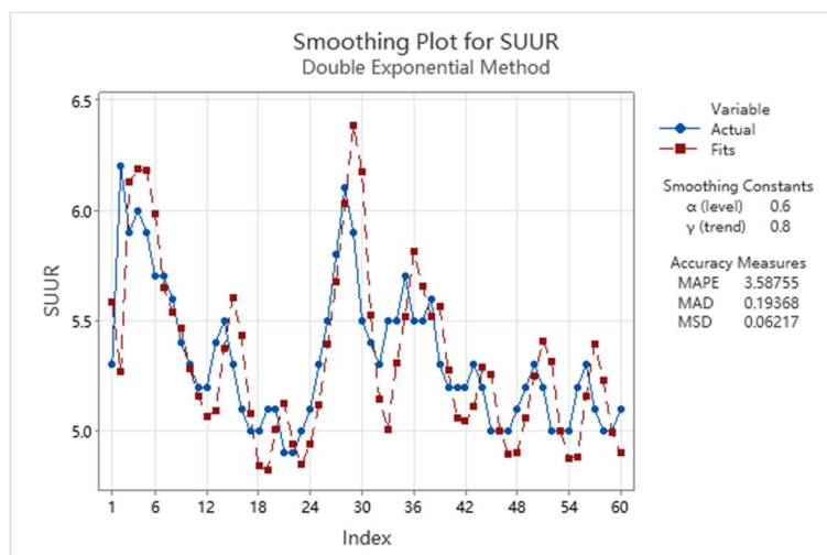
ภาพที่ 9 Double Exponential Method โปรแกรม Minitab 16 ที่มา: Guoxiang (2024)
