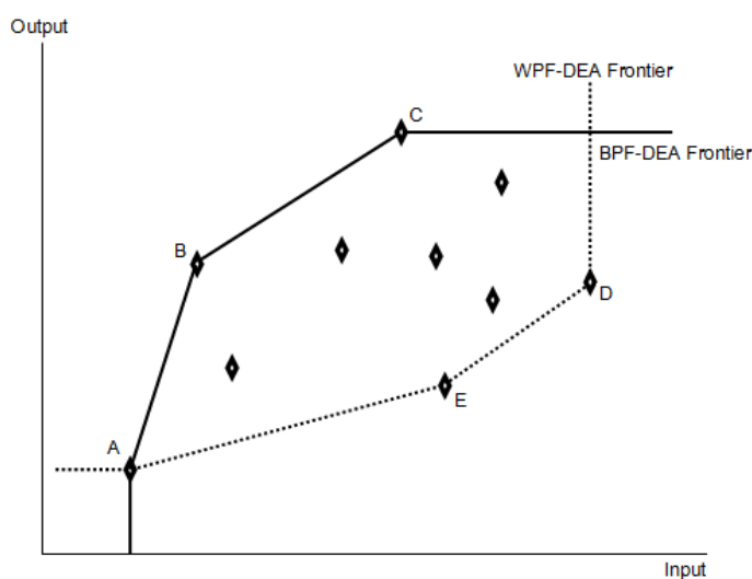
รูปที่ 3 ความแตกต่างของตัวแบบ BPF-DEA และ WPF-DEA
