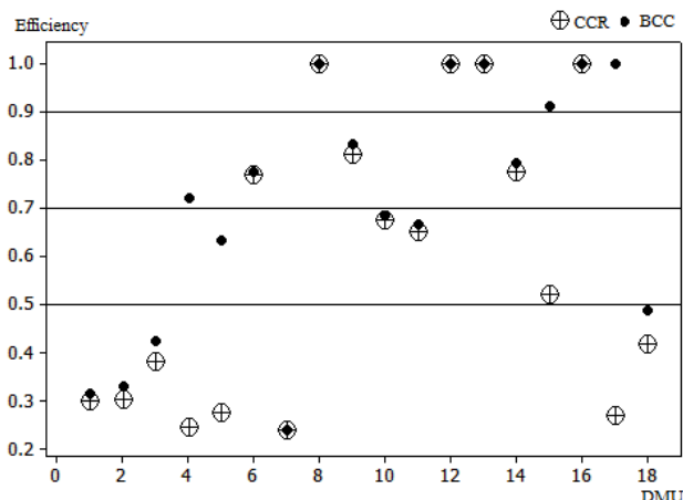
รูปที่ 4 คะแนนประสิทธิภาพของสหกรณ์ในจังหวัดเพชรบุรี จากตัวแบบ CCR และ BCC ของวิธีการ DEA
