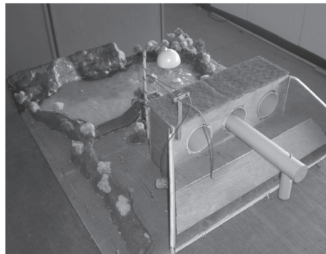
ภาพที่ 6 แบบจำลองพื้นที่และตำแหน่งติดตั้งระบบผลิตไฟฟ้าพลังงานน้ำขนาดเล็กผ่านอุโมงค์ระบายน้ำใต้ถนนบริเวณลำธารสายที่หนึ่ง
