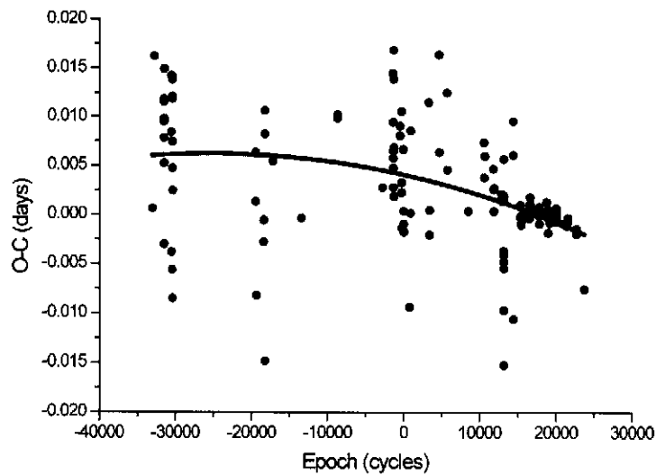
ภาพที่ 4 แผนภาพ O-C ของระบบดาวคู่ CE Leonis
